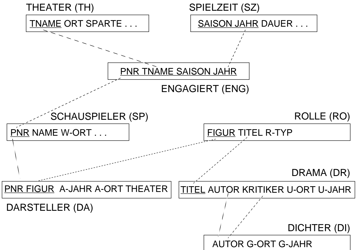
Relationales Schema
