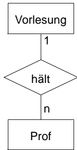
ER-Diagramm
