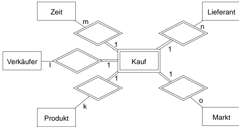
ER-Diagramm
