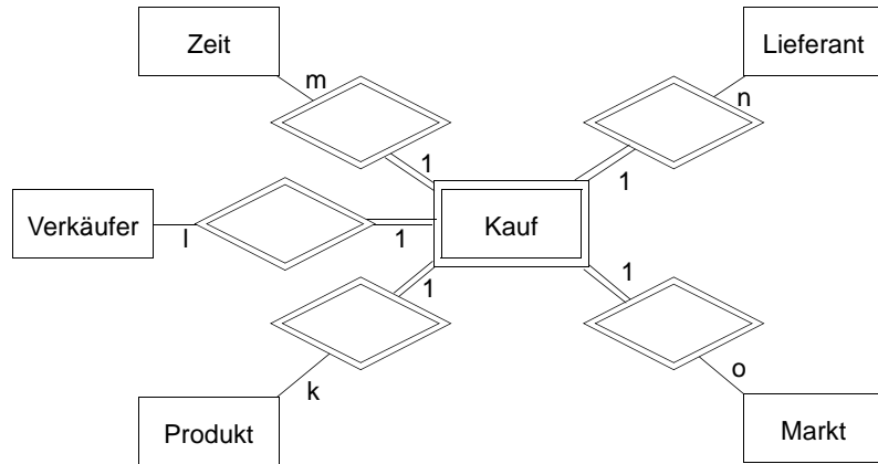
ER-Diagramm
