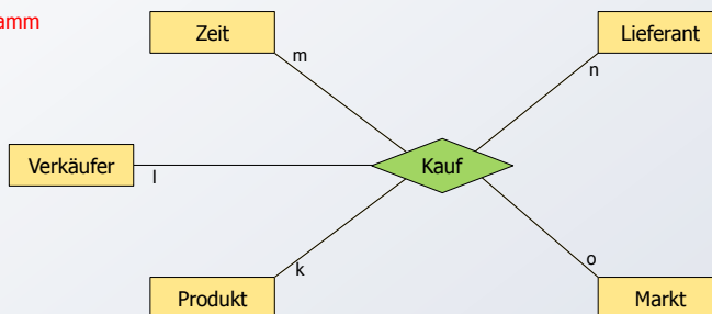
ER-Diagramm
