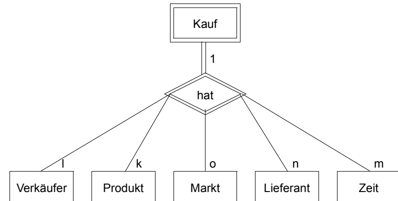
ER-Diagramm
