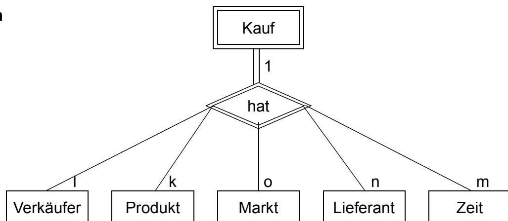
ER-Diagramm
