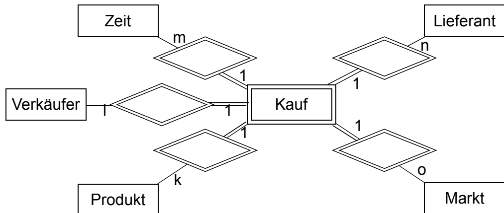
ER-Diagramm
